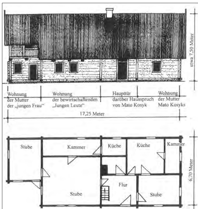
Abb. 9: Der Grundriss des Geburtshauses nach Tetzner. Umzeichnung A. Roggan, aus: Franz Tetzner: Die Slawen in Deutschland. Braunschweig 1902, Abb. 114 „Werbener Wohngebäude“
